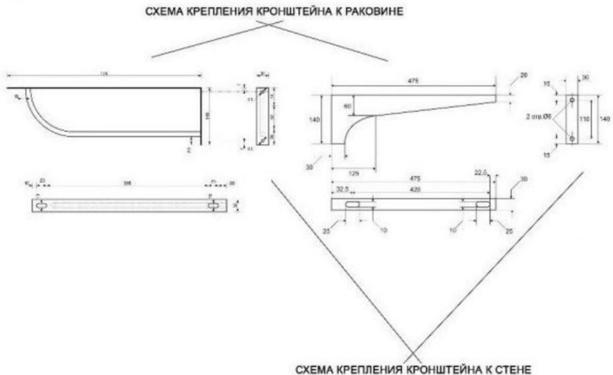
Рис.2 Кронштейн №2 (металл)
